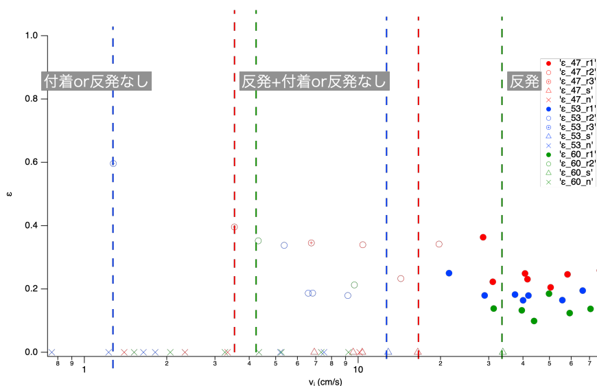
多孔質氷球と多孔質氷板の衝突における衝突速度と反発係数の関係
